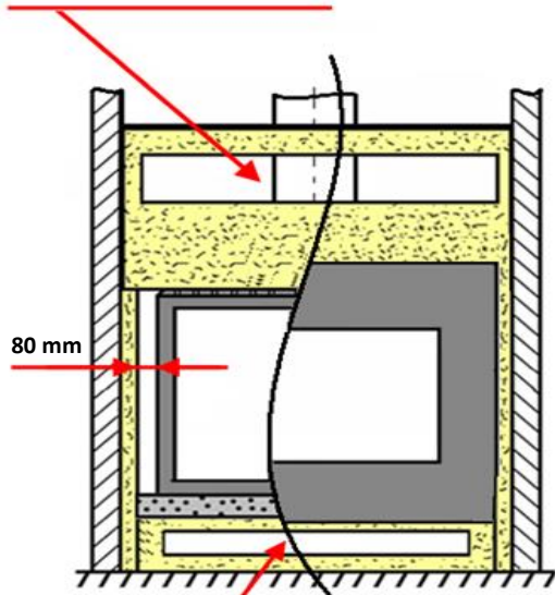
Section de la sortie d'air chaud : 12 dm 2
